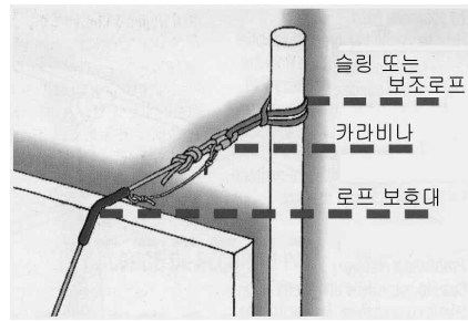
[ 그림 3-50 ] 현수로프의 간접 고정
