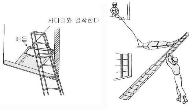
[ 그림 4-21 ] 사다리를 이용한 수평구출 방법
