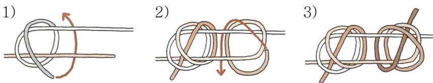
[ 그림 3-18 ] 이중피셔맨매듭
