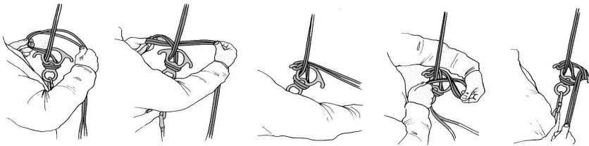
[ 그림 3-80 ] 구조용 하강기를 고정하는 방법
