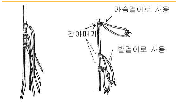
[ 그림 3-91 ] 감아매기 등반 로프 만들기
