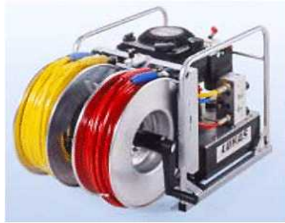
[ 그림 2-29 ] 호스릴이 부착된 유압엔진펌프
