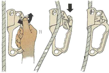
[ 그림 2-10 ] 등강기 사용방법
