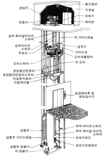
[ 그림 5-101 ] 엘리베이터의 구조
