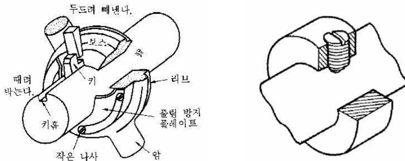
[ 그림 5-9 ] 키와 나사로 고정된 축의 분해방법
