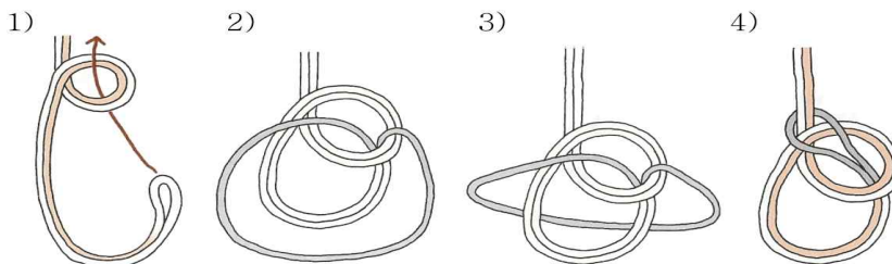
[ 그림 3-10 ] 두겹고정매듭
