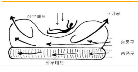
[ 그림 2-37 ] 공기매트의 구조
