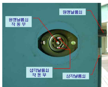
[ 그림 6-2 ] 방화문 잠금장치(내부)
