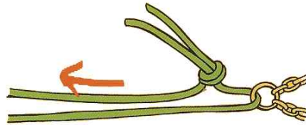
[ 그림 3-52 ] 로프감기 설치방법
