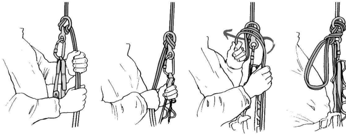
[ 그림 3-79 ] 8자 하강기를 완전히 고정하는 방법
