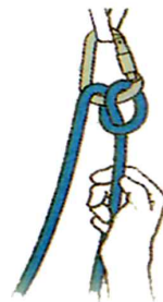
[ 그림 3-71 ] 카라비나와 로프의 마찰력을 이용하는 방법
