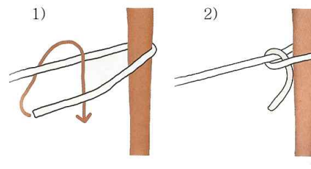
[ 그림 3-21 ] 절반매듭
