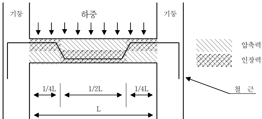
[ 그림 5-83 ] 보의 응력 분포
