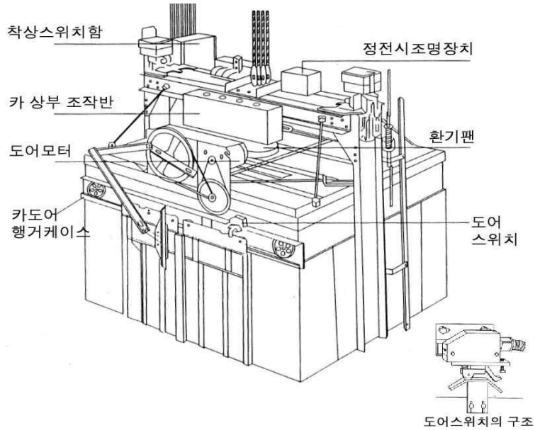
[ 그림 5-102 ] 카 상부의 구조
