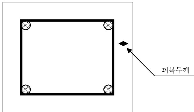
[ 그림 5-85 ] 철근 콘크리트 기둥의 단면도
