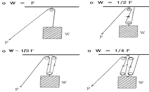
[ 그림 2-12 ] 도르래 숫자와 힘의 이득 관계
