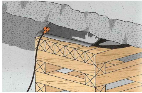
[ 그림 2-28 ] 받침목을 이용한다.
