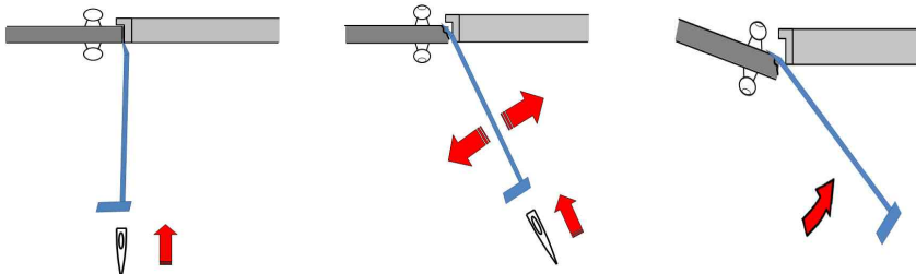
[ 그림 6-23 ] 지렛대 활용 작업(3)
