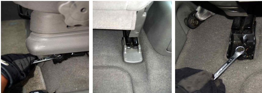
[ 그림 5-34 ] 운전석 의자를 분리하는 방법
