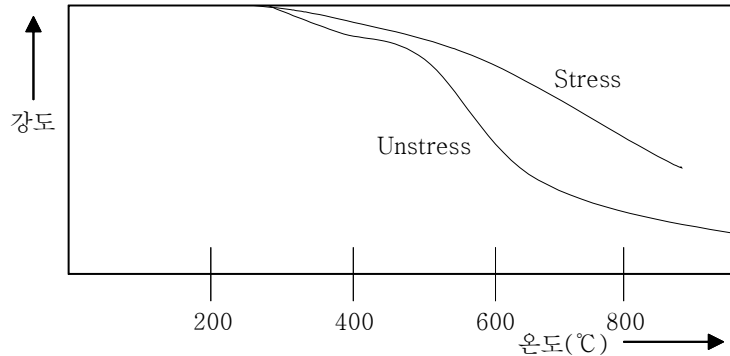
[ 그림 5-84 ] 콘크리트의 온도변화에 따른 강도 변화
