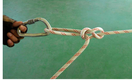
[ 그림 3-57 ] 당김줄매듭을 만들고 카라비나를 건다.
