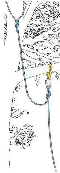
수목을 이용하여 현수로프 설치하는 방법
