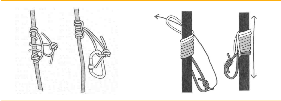
[ 그림 3-24 ] 감아매기(좌)와 클램프하이스트 매듭(우)
