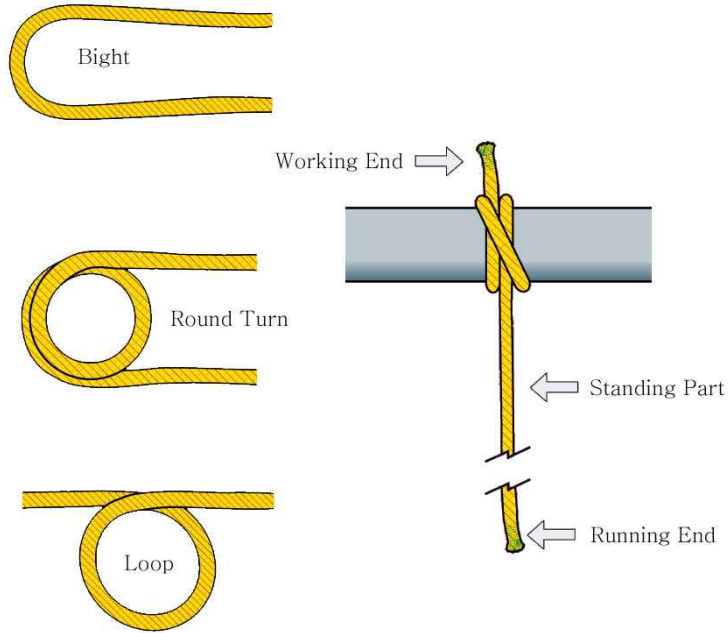
[ 그림 3-1 ] 매듭 각 부분의 명칭
