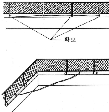
[ 그림 3-46 ] 펜스를 이용하는 방법
