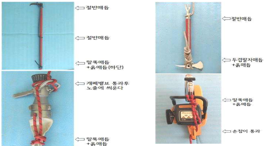
[ 그림 3-29 ] 여러가지 기구 묶기
