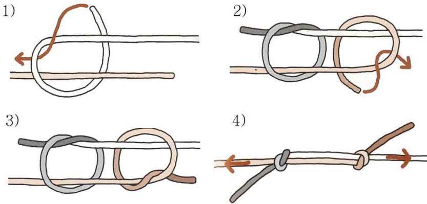
[ 그림 3-18 ] 이중피셔맨매듭
