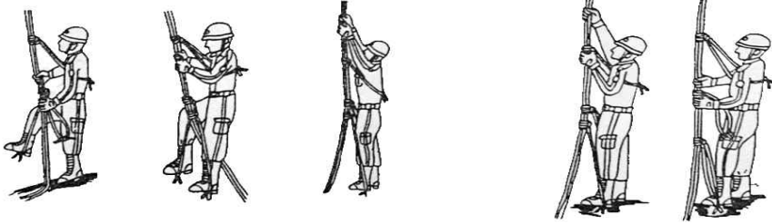
[ 그림 3-92 ] 감아매기 등반 제1(우측), 제2(좌측) 방법
