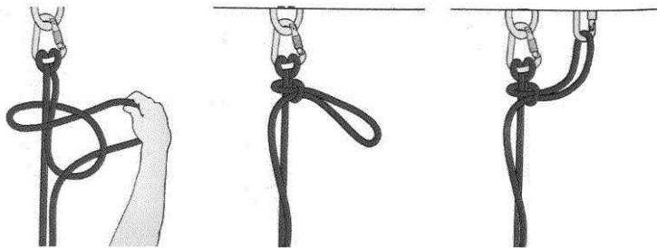
[ 그림 3-51 ] 카라비나에 로프 걸착하기
