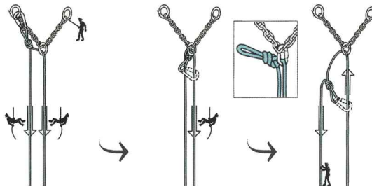
[ 그림 3-53 ] 회수로프 설치방법
