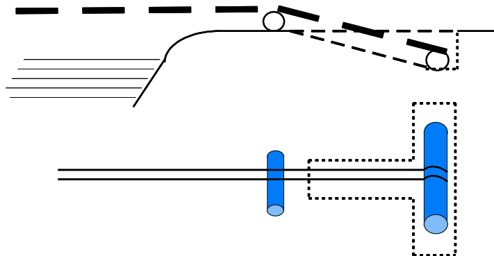
[ 그림 3-43 ] 확보물을 매몰시켜 로프를 설치하는 방법
